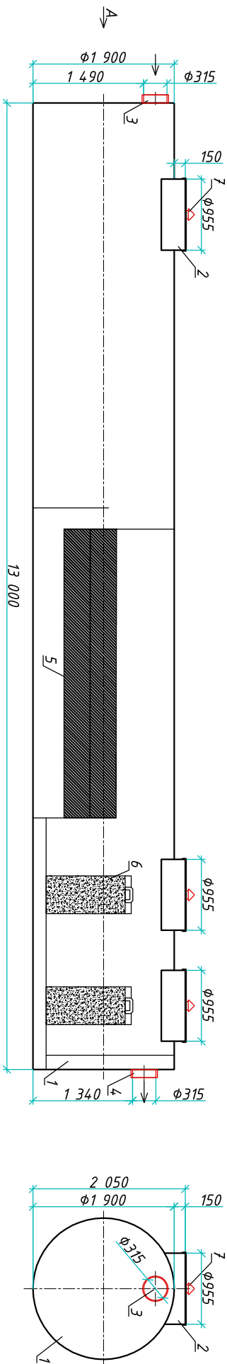
Разрез 1-1
